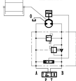
液压原理图
